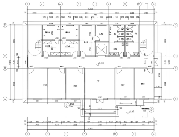
综合楼一层平面图
