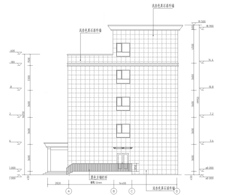
综合楼立面图
