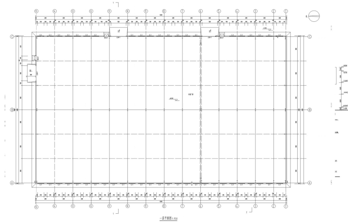
厂房一层平面图
