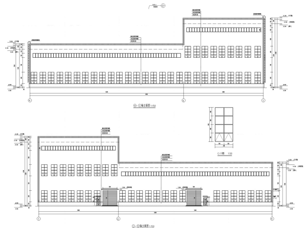
厂房立面图
