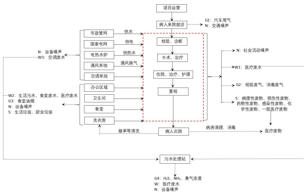
图 2-2 卫生院运营期流程及产污图
