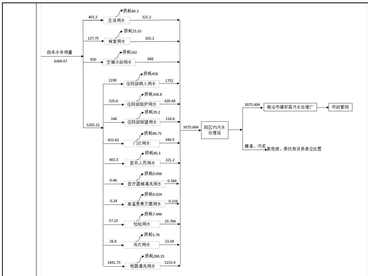
图 2-1 项目水平衡图 (m³/a)
